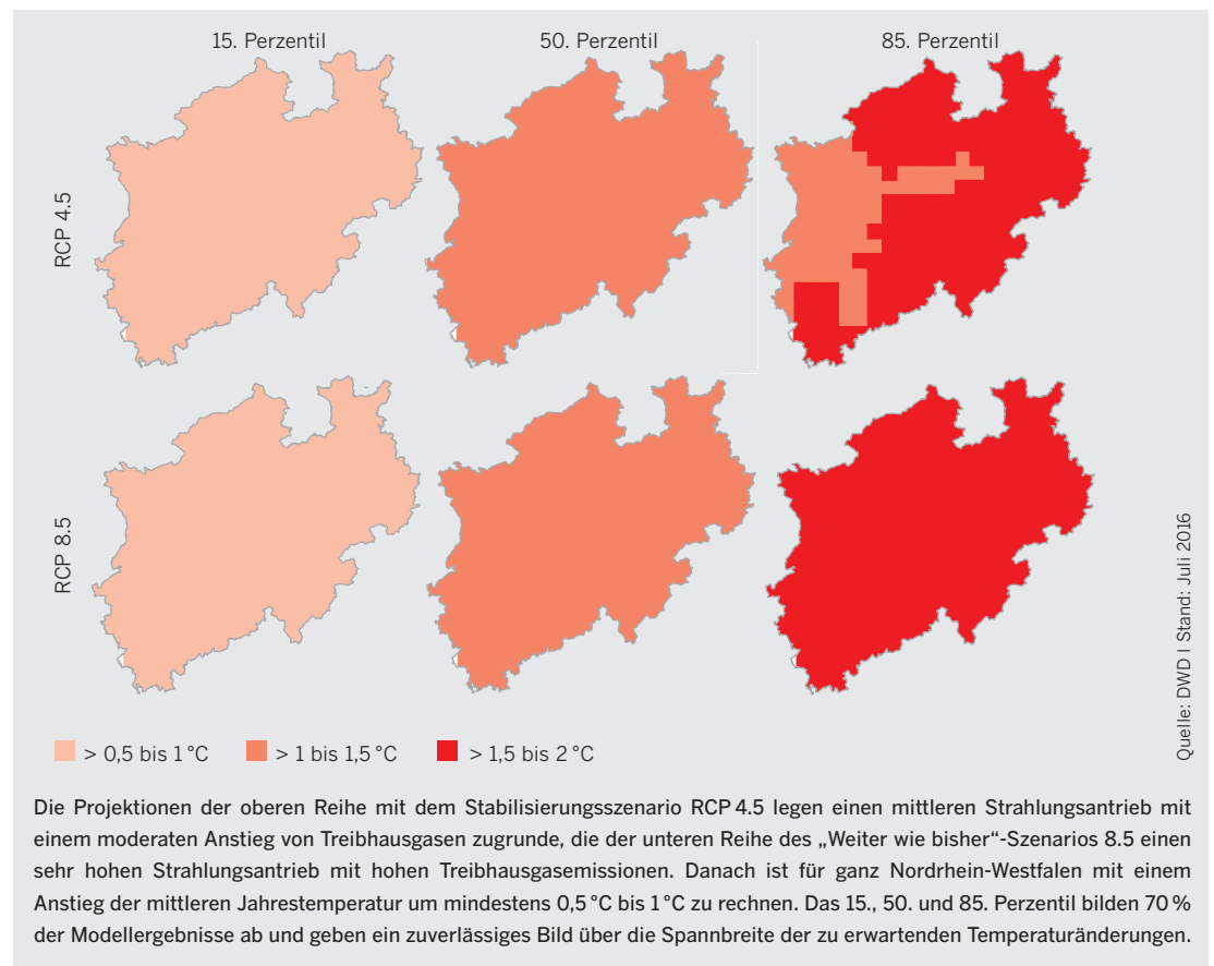
Abbildung 9 Änderung der mittleren jährlichen Lufttemperatur 2021 bis 2050 bezogen auf 1971 bis 2000 in NRW
