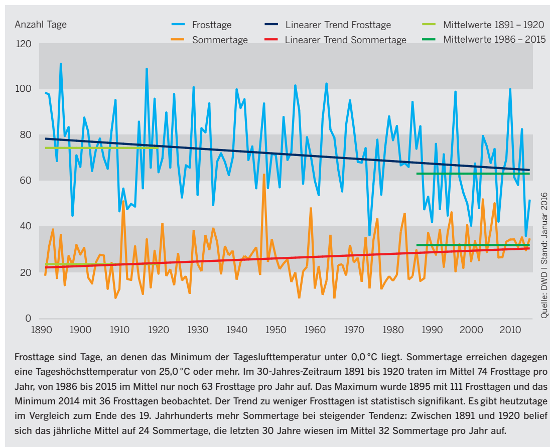
Abbildung 16 Frost- und Sommertage in NRW
