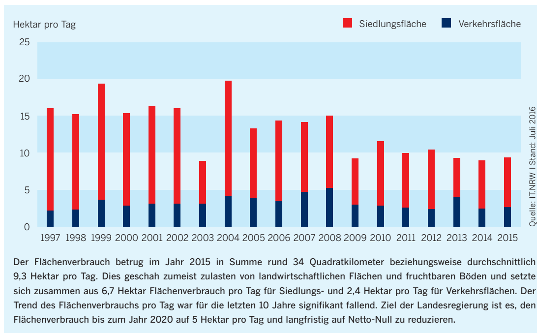
Abbildung 49 Umweltindikator Flächenverbrauch in NRW Teilindikator Zunahme der Siedlungs- und Verkehrsfläche
