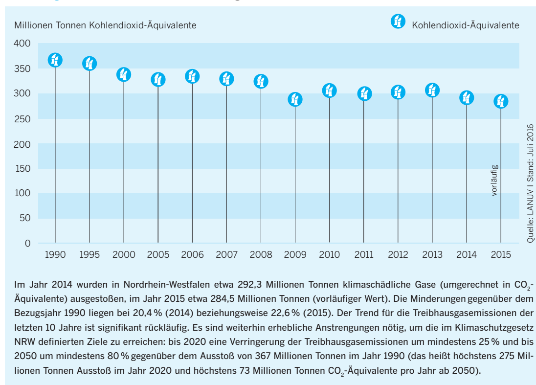
Abbildung 21 Umweltindikator Treibhausgasemissionen in NRW
